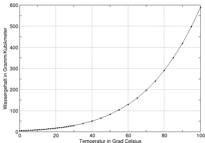
Saettigungsmenge von Wasserdampf in der Luft
